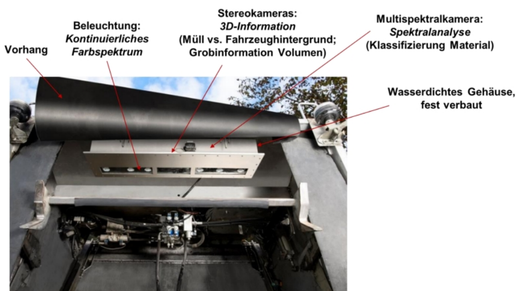
Abbildung 4: Hardware des Grüngutscanners, Quelle: Contena-Ochsner & Biomasse Suisse, 2019, PowerPoint-Präsentation Grüngutscanner, S. 4
